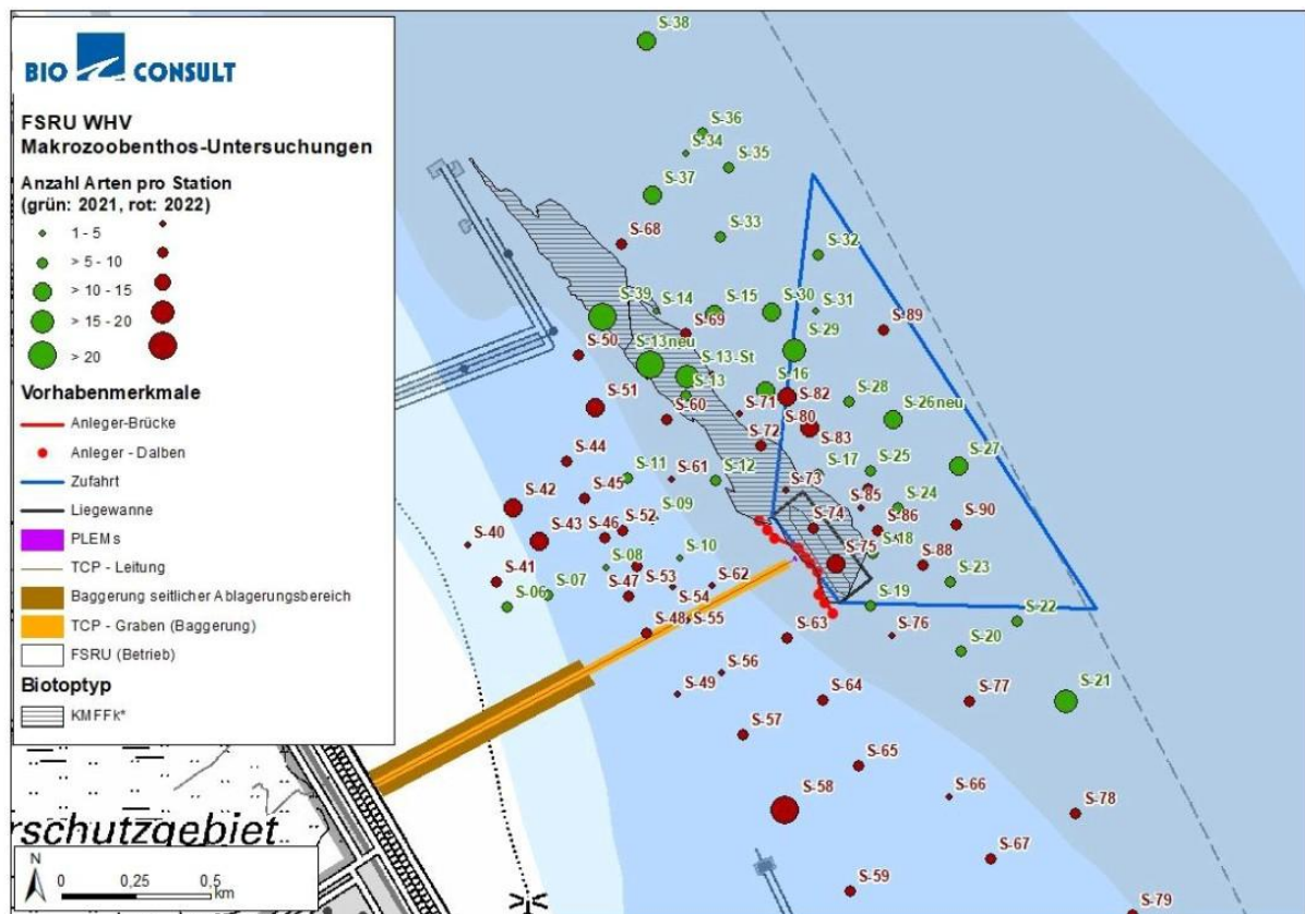
Abbildung 27: Stationsraster der Benthosbeprobungen und räumliche Visualisierung der Gesamtartenzahl (5 Klassen) der Beprobungen in 2021 und 2022 (Quelle: BioConsult 2023b)
