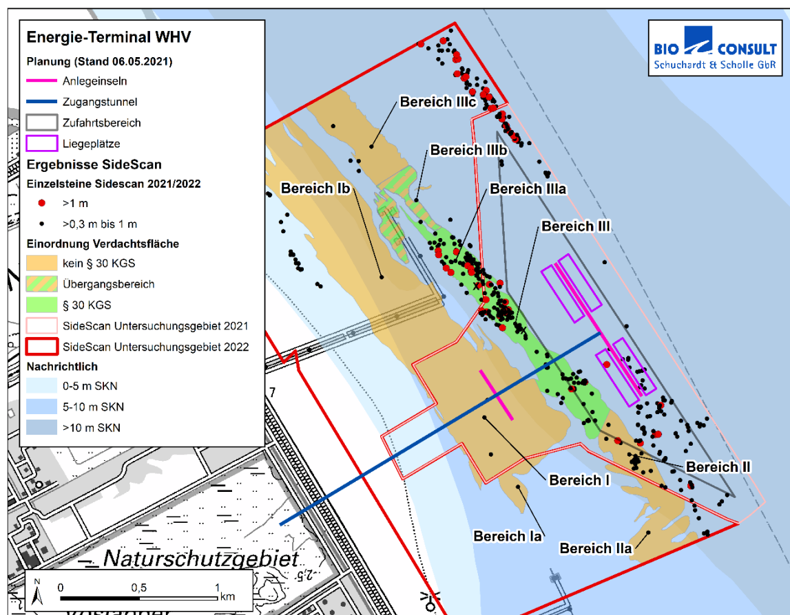
Abbildung 28: Vorkommen des nach § 30 BNatSchG geschützten Biotoptyps „artenreiche Kies-, Grobsand- und Schillgründe“ im Untersuchungsgebiet 2021/2022 (Quelle: BioConsult GmbH & Co. KG 2022)
